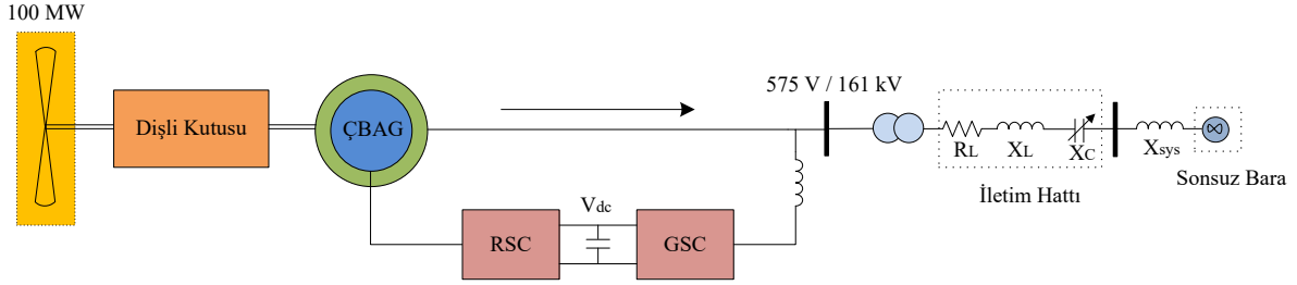
Şekil 3. Bu çalışmada oluşturulan benzetim çalışması
