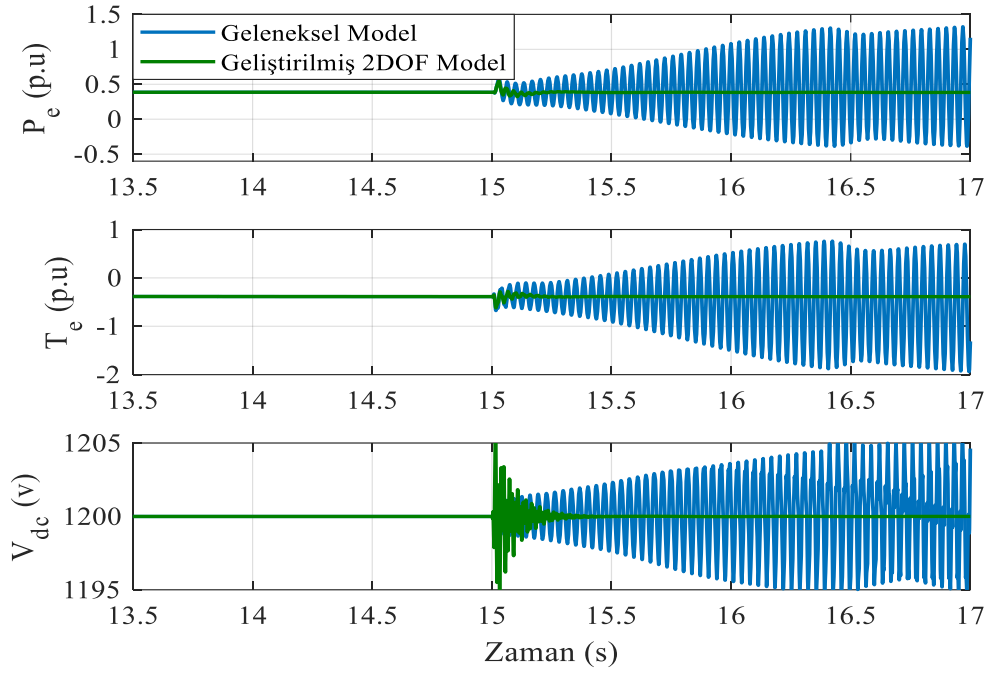
Şekil 4. 9 m/s rüzgar hızı ve kompanzasyon oranı %50 iken elde edilen sonuçlar
