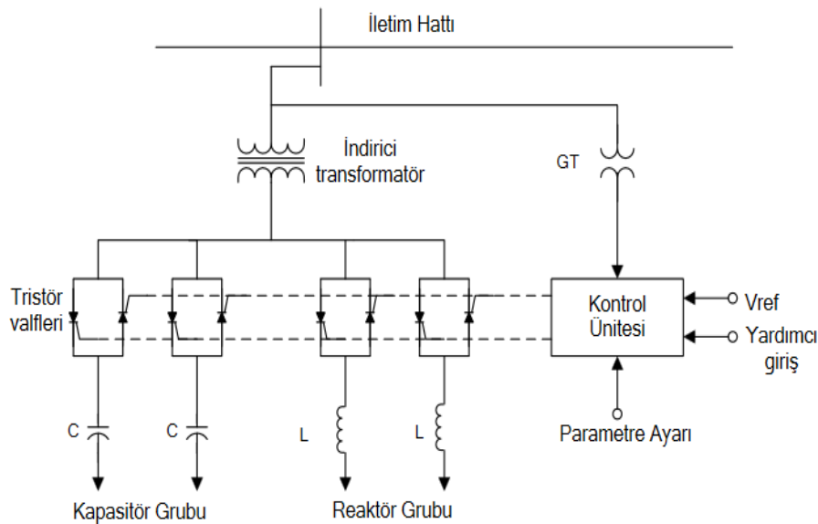
Şekil 1. SVC modeli.
