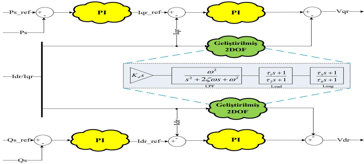
Şekil 2. Geliştirilen 2DOF yapısı
