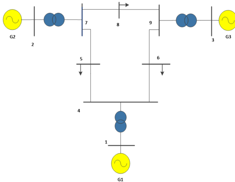
Şekil 2. 9 baralı test sistemi.
