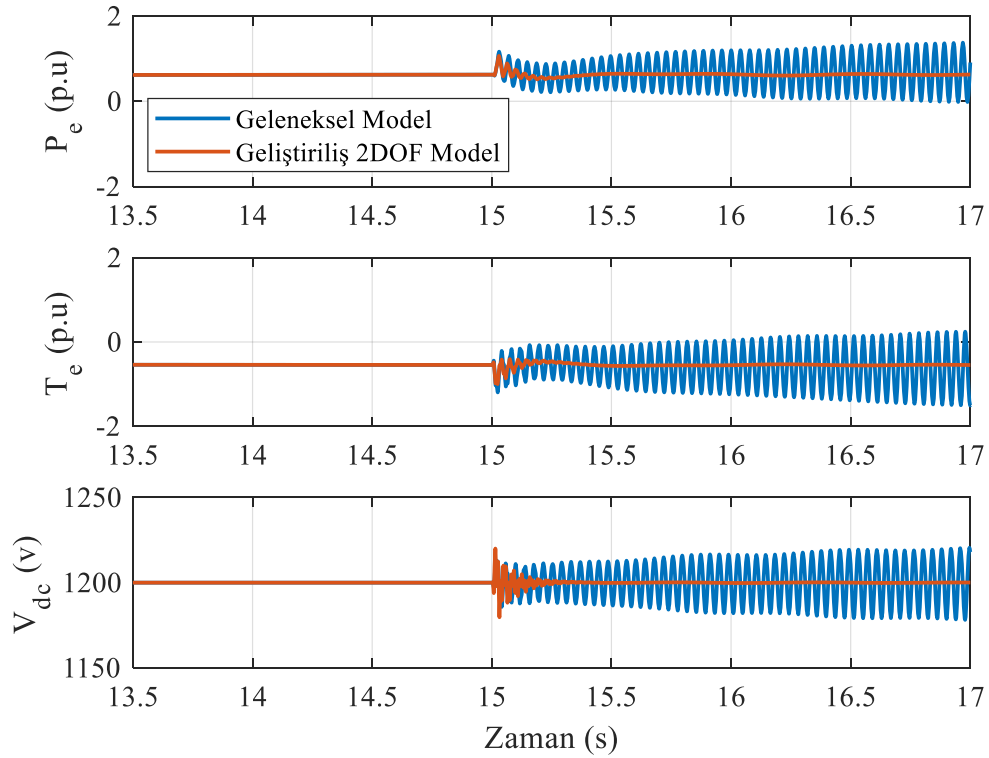
Şekil 7. 11 m/s rüzgar hızı ve kompanzasyon oranı %60 iken elde edilen sonuçlar
