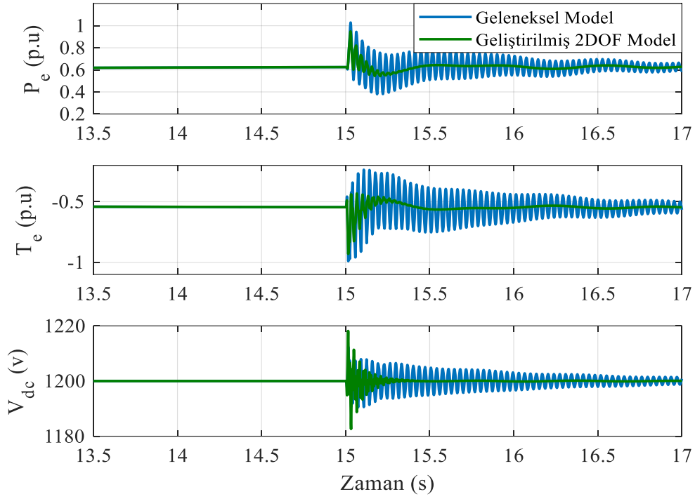
Şekil 6. 11 m/s rüzgar hızı ve kompanzasyon oranı %50 iken elde edilen sonuçlar
