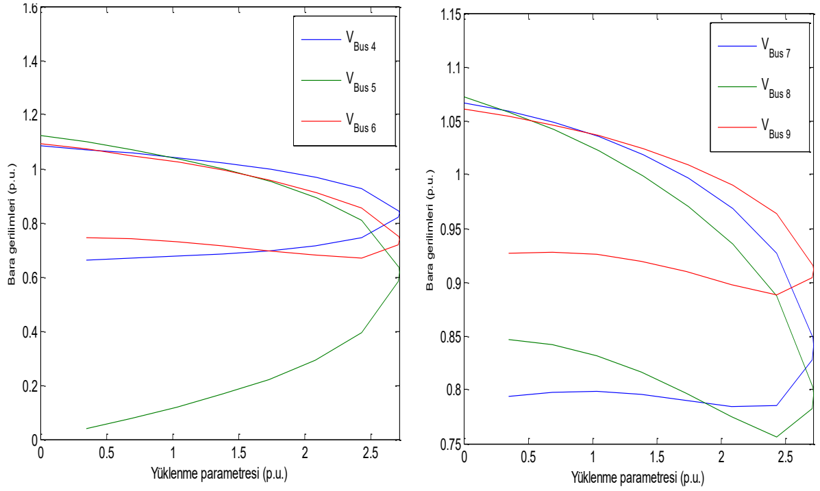
Şekil 4. STATCON'un kullanıldığı durumdaki sonuçlar.
