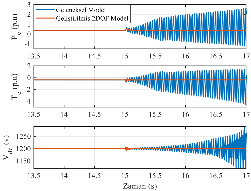
Şekil 5. 9 m/s rüzgar hızı ve kompanzasyon oranı %60 iken elde edilen sonuçlar
