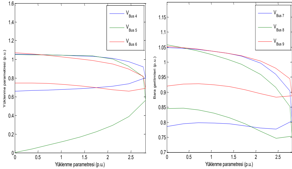
Şekil 5. STATCON ve SVC'nin birlikte kullanıldığı durumdaki sonuçlar.
