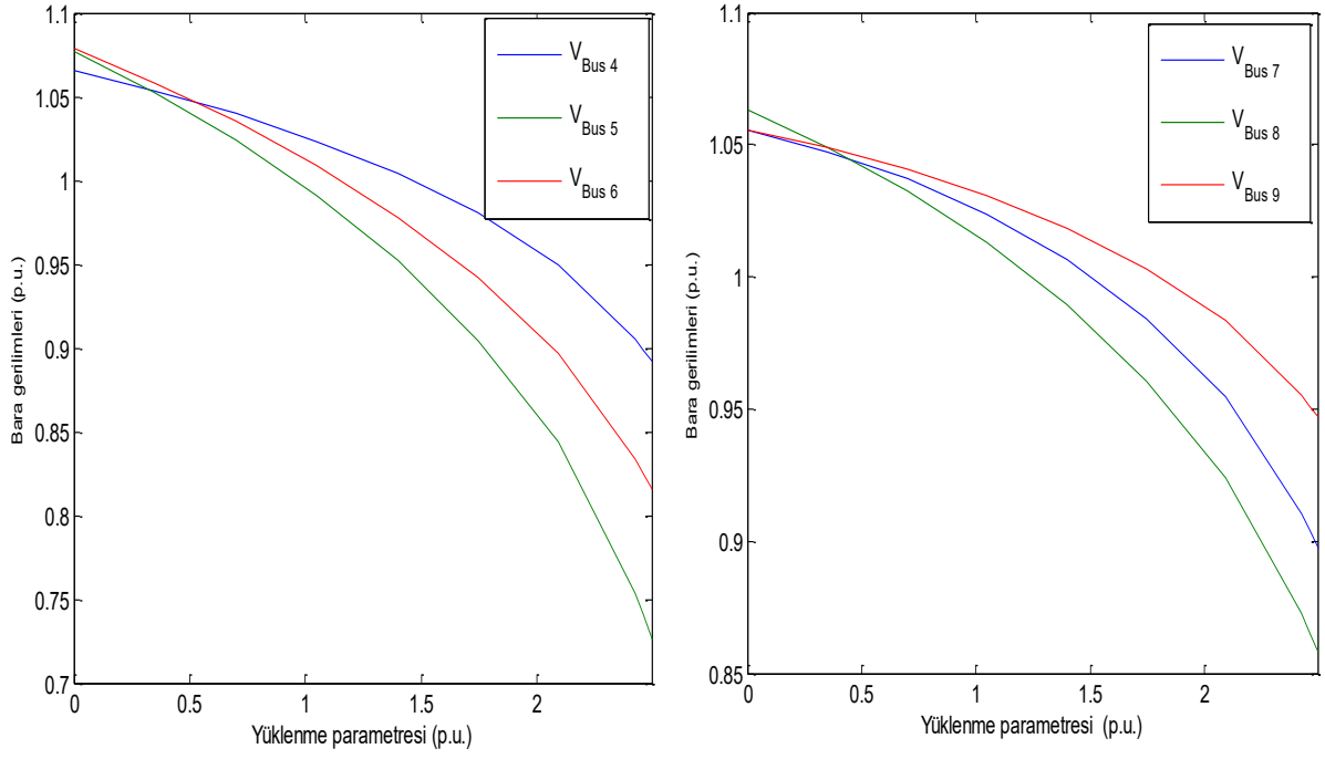
Şekil 3. STATCON ve SVC'nin kullanılmadığı durumdaki sonuçlar.
